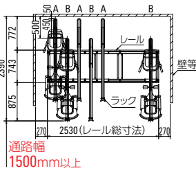
基礎平面図
