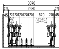
正面図
