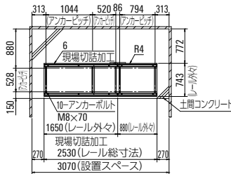
基礎平面図
