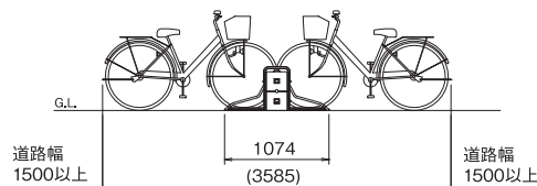
〈RW6/RW12側面図〉
