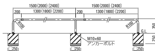
■基礎ベース式
